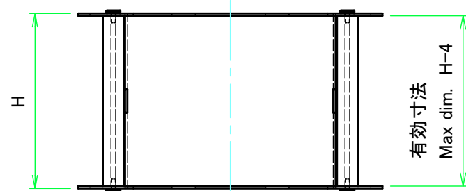
Wパネル1 / W panel 1
